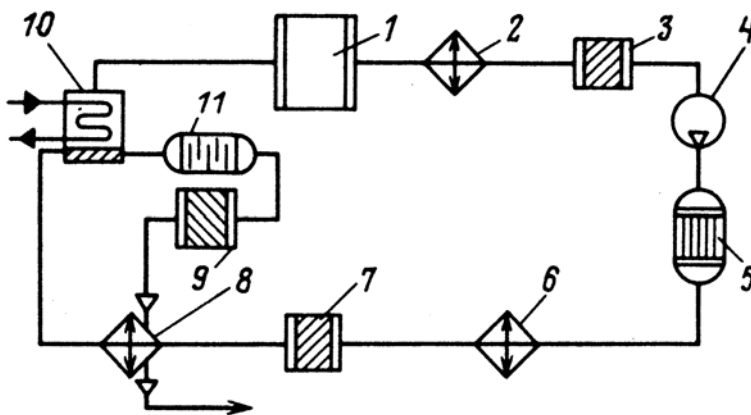
Рис.17 Принципиальная схема газового контура РБМК: 1 – реактор, 2 – теплообменник; 3 – иодный фильтр; 4 – компрессор; 5 – контактный аппарат; 6 – конденсатор; 7 – цеолитовый адсорбер; 8 – газохладитель; 9 – угольный адсорбер; 10 – дефлегматор; 11 – сосуд выдержки.
