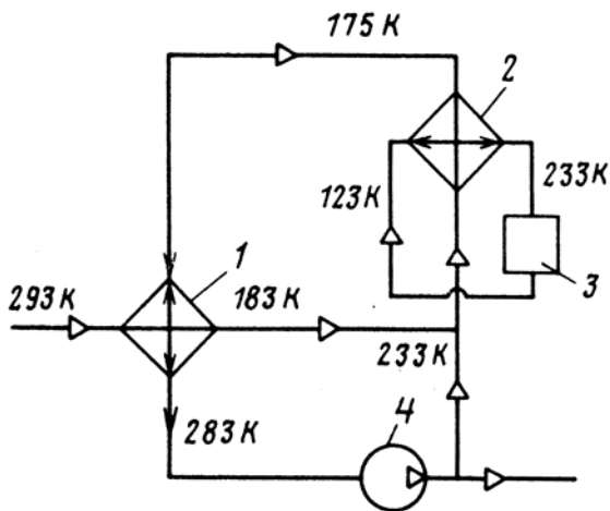
Рис.11 Регенеративная схема вымораживания с рециркуляцией газа
